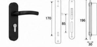
DETALLE CHAPA ESC 1:2
