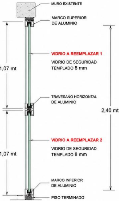
DETALLE MARCO DE ALUMINIO ESC. 1:2
