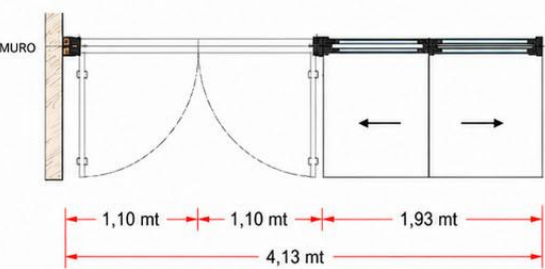
PLANTA ESC 1:25
