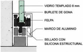
DETALLE MARCO DE ALUMINIO ESC. 1:2
